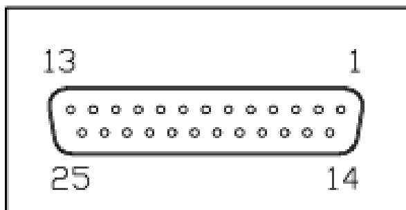
<D-SUB 25 «розетка» RS-232>
